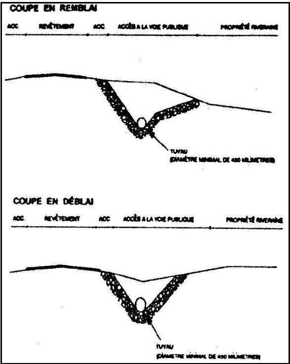
Figure 9.2 Côtés latéraux de l'accès
