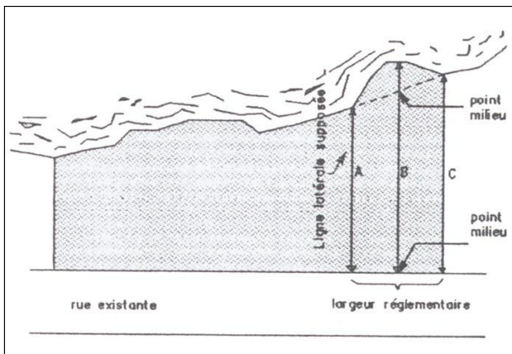
Figure 2. 8 Largeur moyenne d'un lot irrégulier
