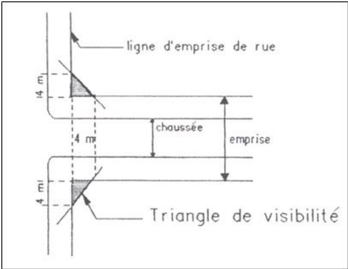
Figure 7. 1 Triangle de visibilité
