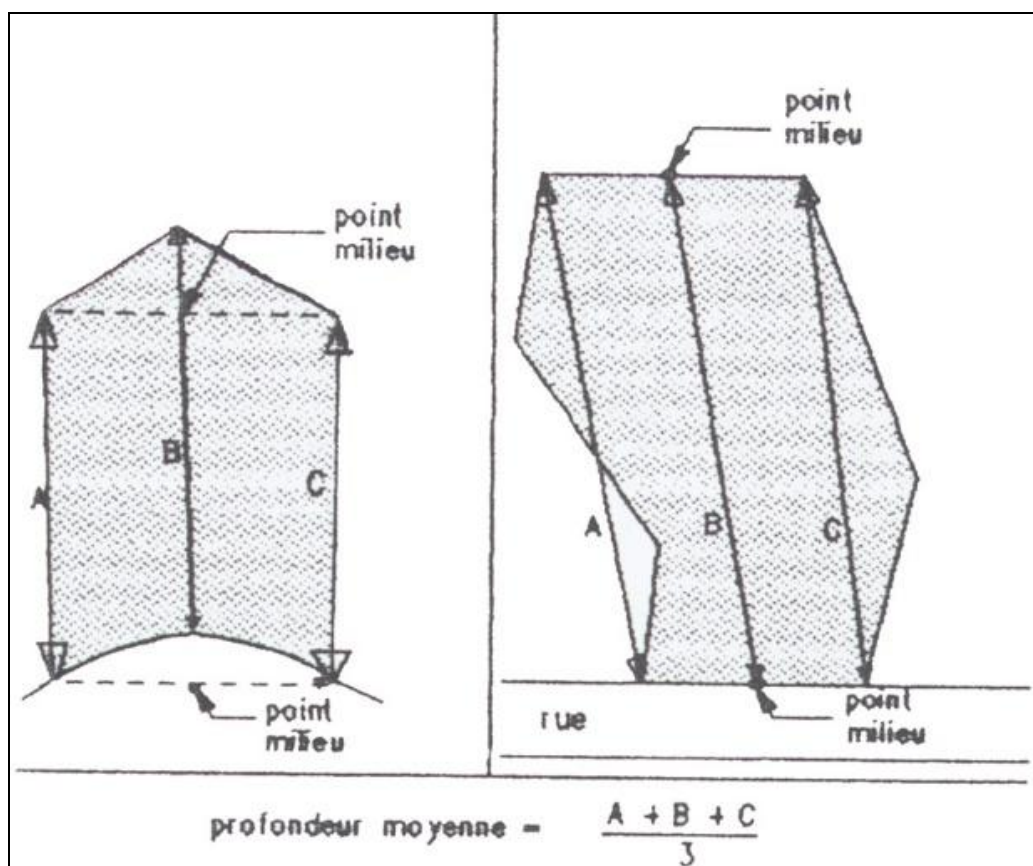
Figure 2. 7 Profondeur moyenne d'un lot irrégulier
