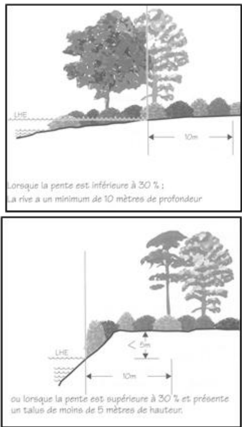
Figure 10.1 : Rive de 10 mètres de profondeur
